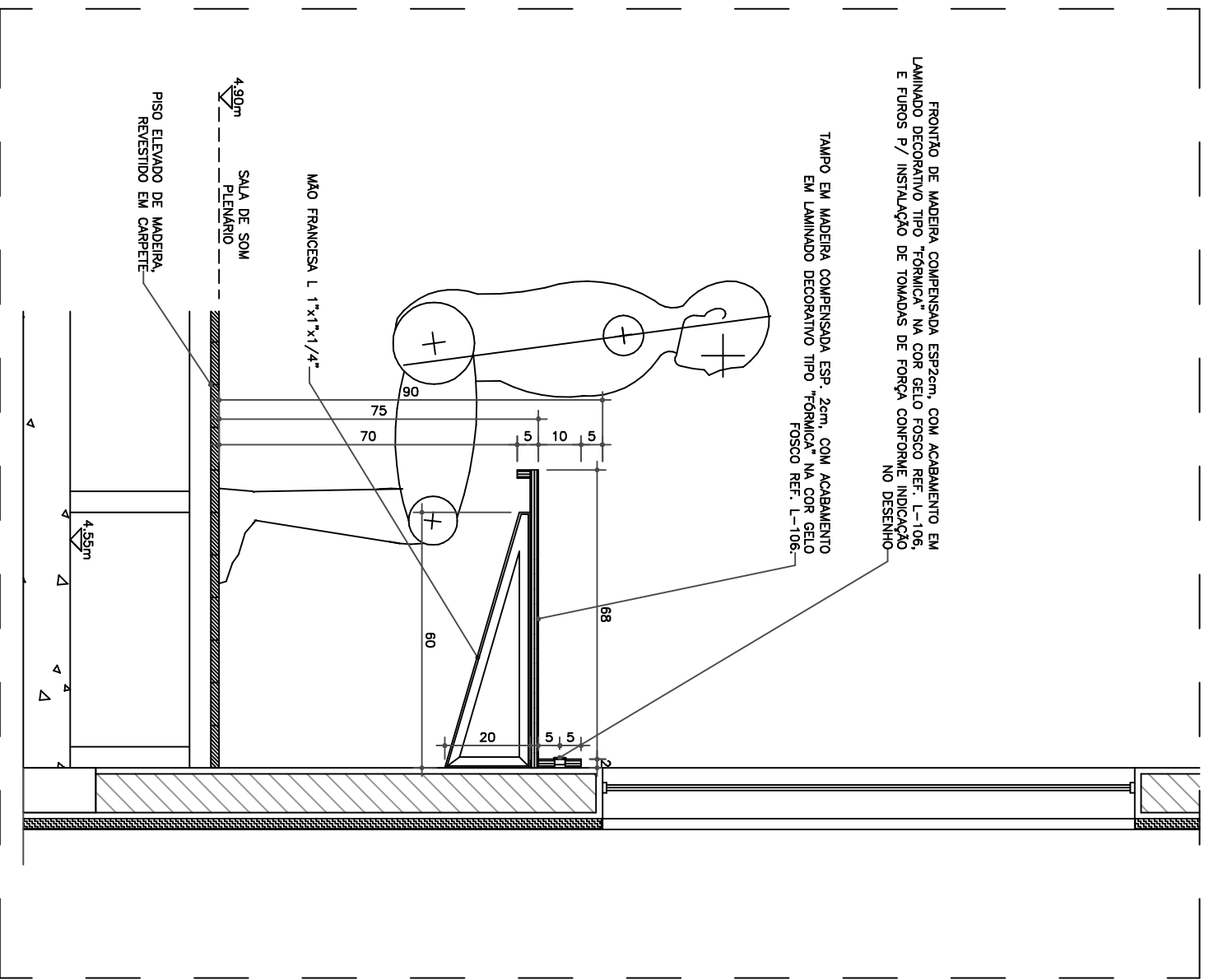
CORTE D ESCALA 1:10 MEDIDAS EM CENTÍMETROS SEÇÃO TRANSVERSAL NA BANCADA DA SALA DE SOM DO PLENÁRIO NO TÉRREO SUPERIOR
