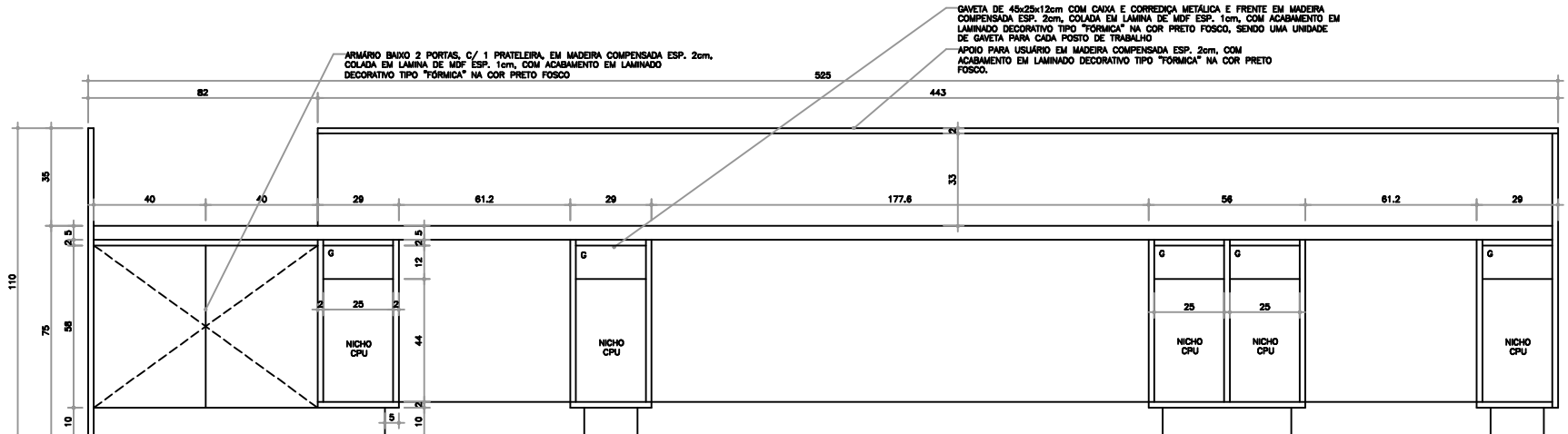
ELEVAÇÃO 1 ESCALA 1:10 MEDIDAS EM CENTIMETROS VISTA POSTERIOR DO BALCÃO DE ATENDIMENTO DA OUVIDORIA NO TERREO INFERIOR
