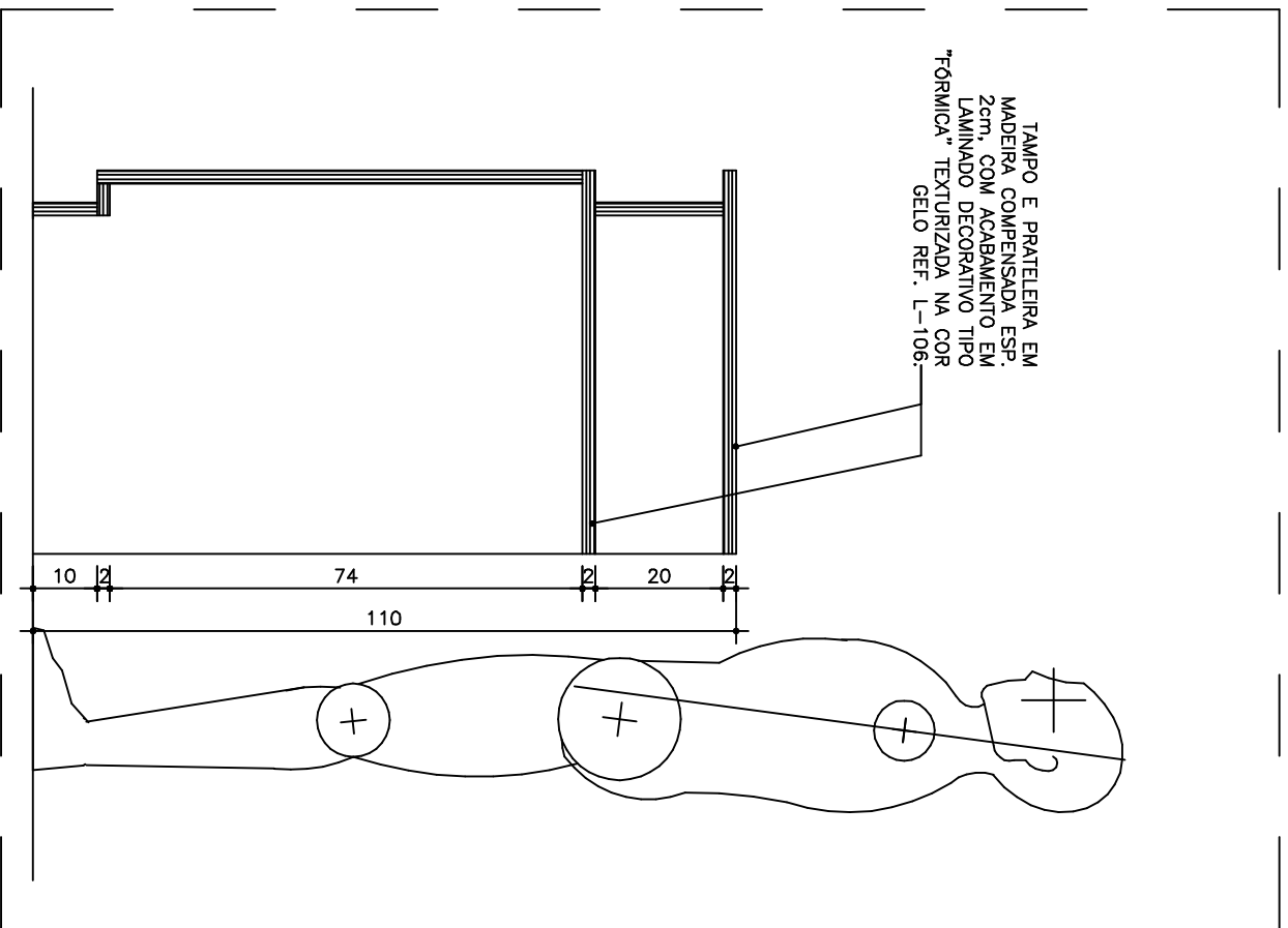
CORTE AA ESCALA 1:10 MEDIDAS EM CENTIMETROS 16 UNIDADES BALÇÃO
