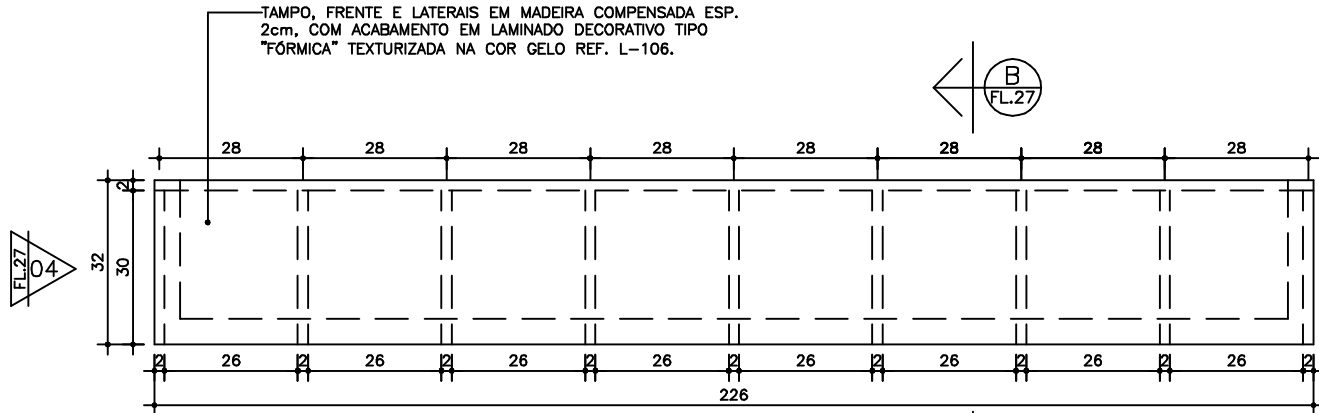
PLANTA ESCALA 1:10 MEDIDAS EM CENTIMETROS 01 UNIDADE ESCANINHO DA REVISÃO DA TAQUIGRAFIA - 40 REPARTIÇÕES
