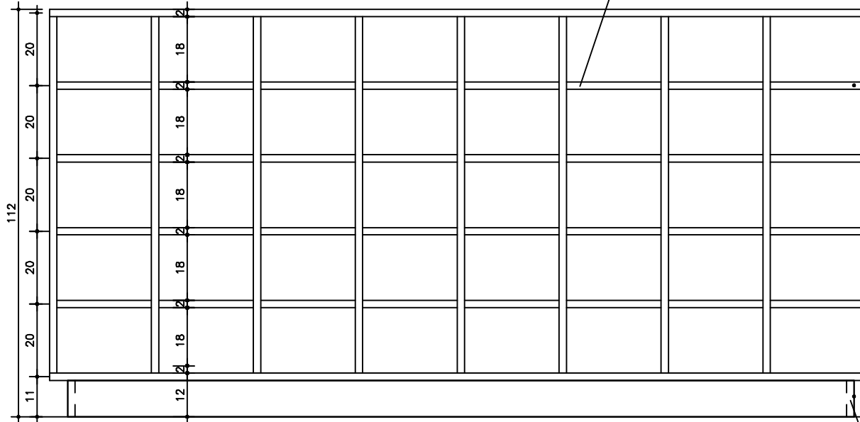
ELEVÇÃO 03 ESCALA 1:10 MEDIDAS EM CENTIMETROS 01 UNIDADE ESCANINHO DA REVISÃO DA TAQUIGRAFIA - 40 REPARTIÇÕES
