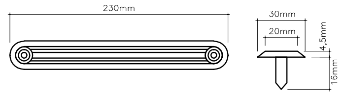
DETALHE_piso tátil direcional
