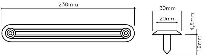
DETALHE_piso tátil direcional
