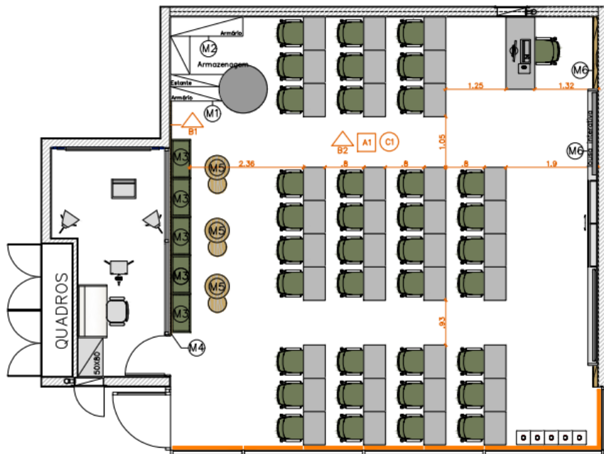
1 Layout com mobiliário - Variação 01 ESCALA 1:75
