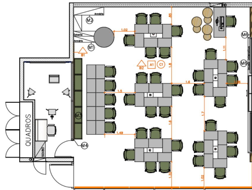
1 Layout com mobiliário - Variação 02 ESCALA 1:75
