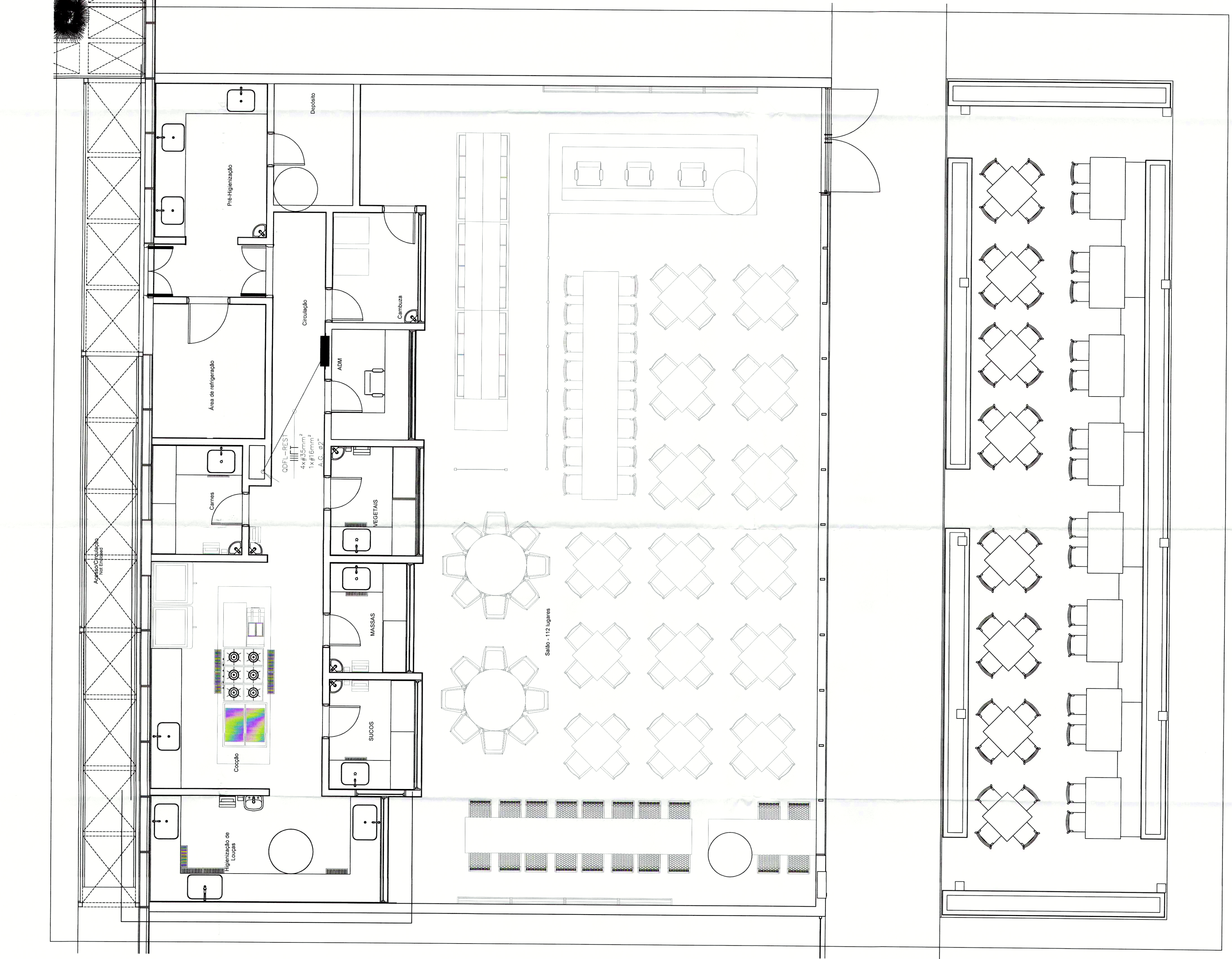
PLANTA BAIXA ELÉTRICA - ALIMENTADOR QUADRO DE LUZ ESC.:1/50
