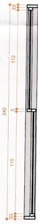
Planta Baixa . J-03
