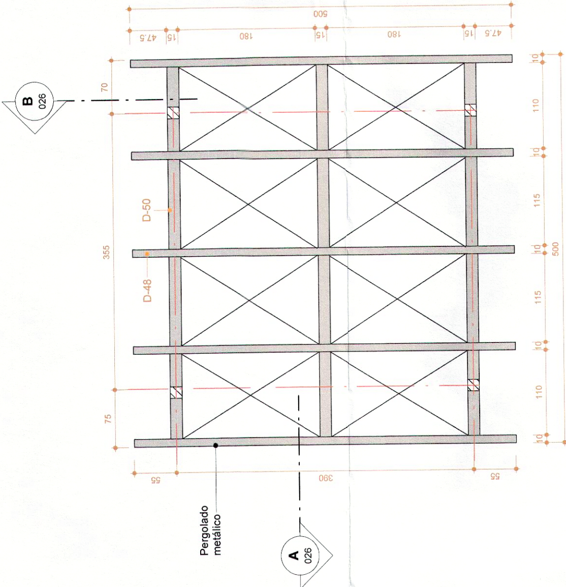
Planta Baixa . Pergolado . Praça 1 : 50
