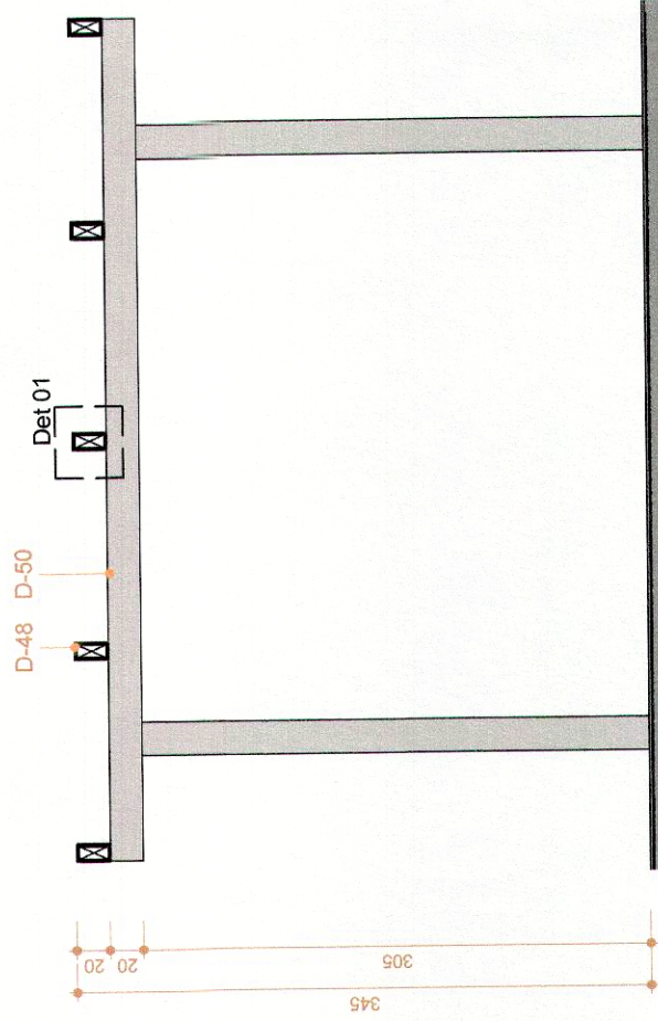
Corte AA . Pergolado Praça 1 : 50
