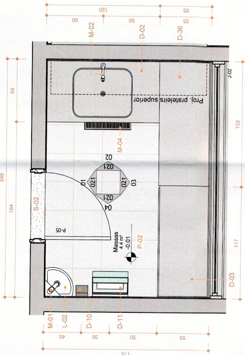
Planta Baixa. Massas 1 : 25
