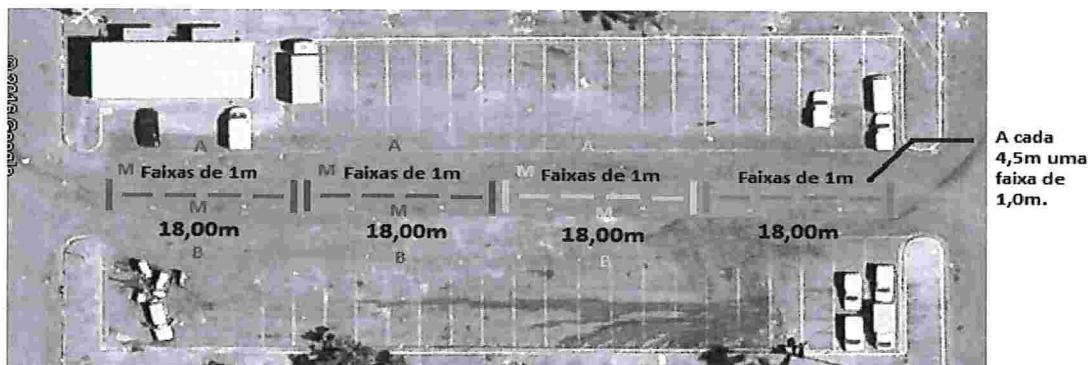
Figura 3: (sinalização no pavimento utilizando cores)
